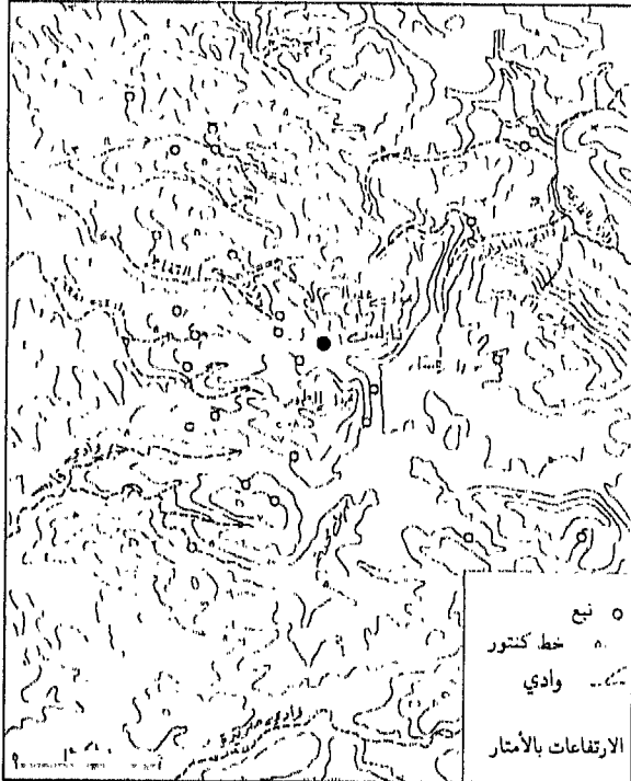
مناسيب سطح الأرض لمنطقة نابلس ( عن خرائط دائرة الأراضي والمساحة الأردنية لوحة نابلس مقياس : ١٠٠,٠٠٠ )
